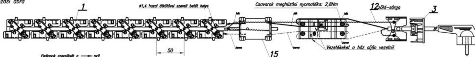
Huzalozási ábra
